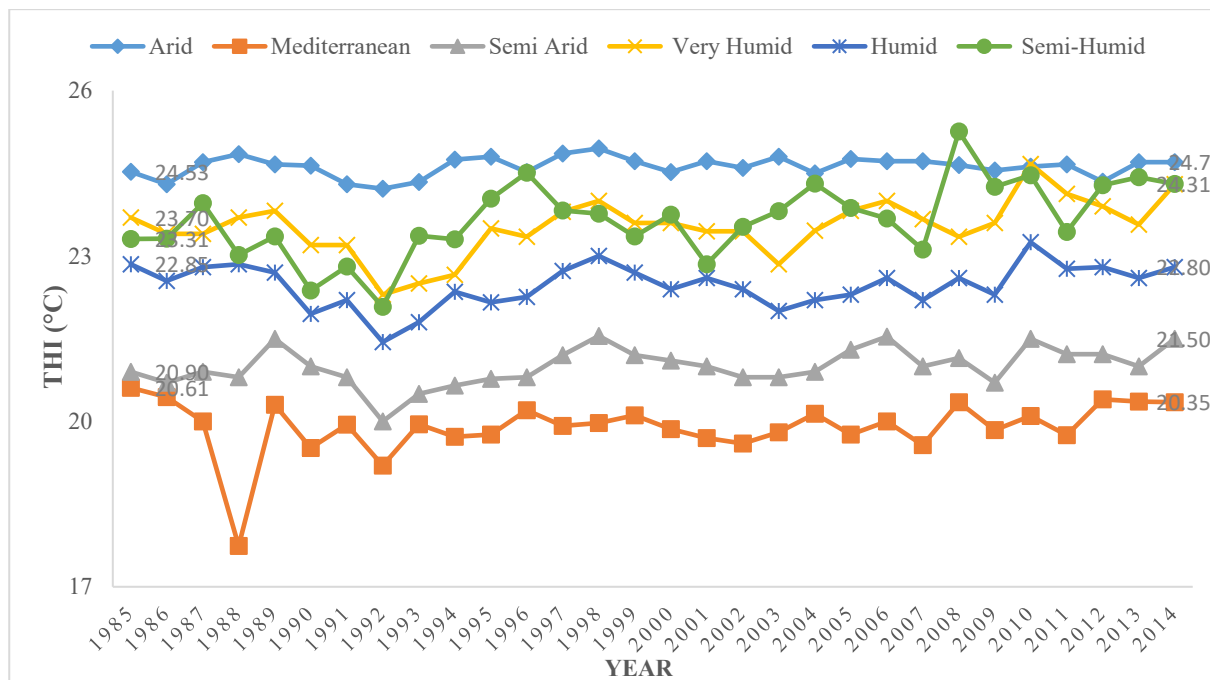
شکل ۳. نمودار تغییرات شاخص THI برای اقلیم‌های مختلف کشور طی دوره ۳۰ ساله در فصل تابستان
