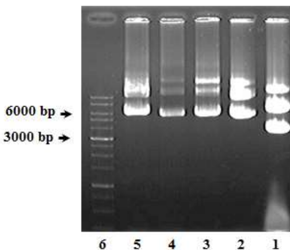
شکل ۷. مقایسه الگوی حرکتی پلاسمیدهای نو ترکیب pcDNA3-hFIX-EGFP با پلاسمید pcDNA3.1 بر روی ژل آگارز ۱٪. ستون ۱: پلاسمید pcDNA3.1، ستون ۲ تا ۵: پلاسمیدهای نو ترکیب pcDNA3-hFIX-EGFP، ستون ۶: نشانگر وزن مولکولی DNA (1 kb).
