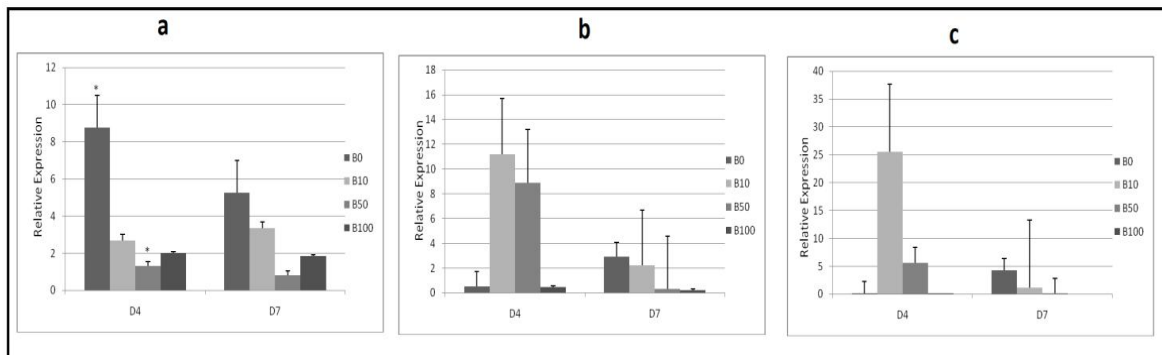
نمودار ۳: مقایسه بیان نسبی ژن های مورد ارزیابی بوسیله Real Time PCR که به مدت ۴ و ۷ روز در معرض غلظت های مختلف BMP4 قرار گرفته اند. بیان نسبی Oct4 نسبت به \beta -actin (a)، Stella نسبت به \beta -actin (b) و Mvh نسبت به \beta -actin (c)
