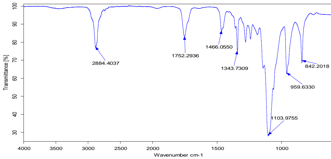
شکل ۶- طیف FT-IR کوپلیمر mPEG-PCL
