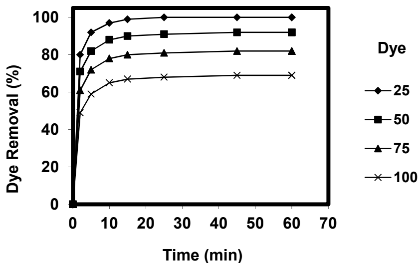
شکل ۵: اثر غلظت رنگزا بر راندمان حذف رنگزای اسید بلاک ۱ توسط جاذب کامپوزیت نانولوله‌های کربنی- دندریمر (مقدار جاذب ۰/۱ گرم در لیتر و سرعت همزن ۲۰۰ دور در دقیقه).
