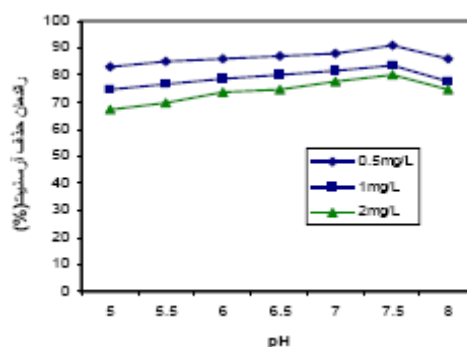
شکل ۱۵: تأثیر pH بر راندمان حذف آرسنات
