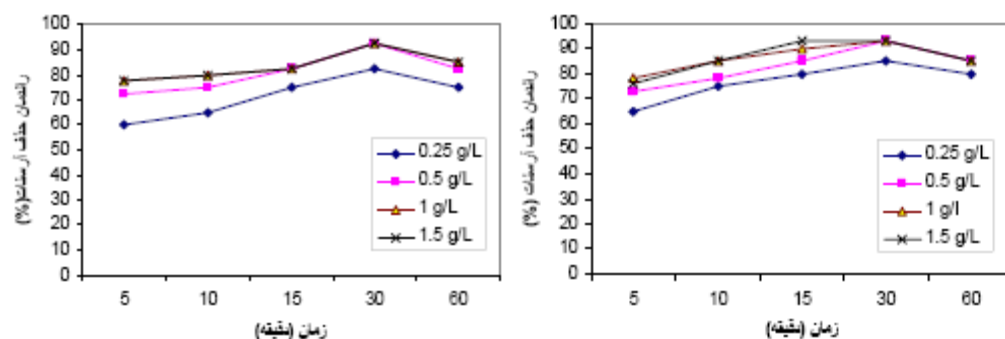
شکل ۱: تأثیر زمان بر راندمان حذف آرسنات در غلظت اولیه ۰/۵ mg/L. شکل ۲: تأثیر زمان بر راندمان حذف آرسنات در غلظت اولیه ۱ mg/L
