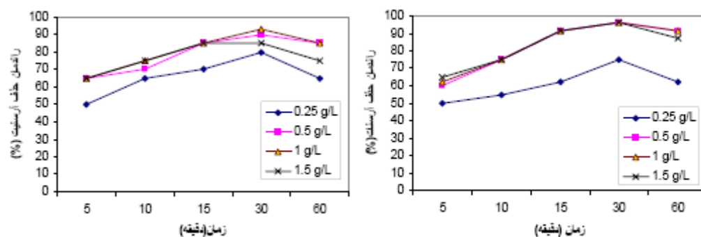
شکل ۳: تأثیر زمان بر راندمان حذف آرسنات در غلظت اولیه ۲ mg/L. شکل ۴: تأثیر زمان بر راندمان حذف آرسنیت در غلظت اولیه ۰/۵ mg/L
