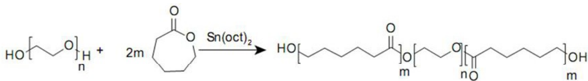
شکل ۱- مسیر سنتز کوپلیمر PCL-PEG-PCL
