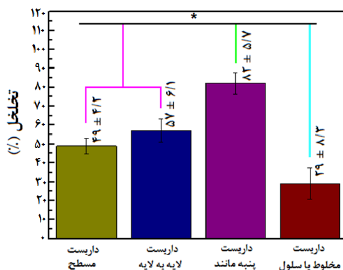
شکل ۹. نمودار تخلخل الیاف PCL/ G/ PDMS با مورفولوژی‌های مختلف. نتایج به صورت میانگین ( P < 0.05 ) \pm SD بیان شده است.
