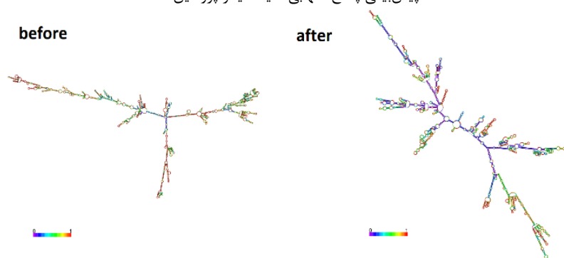
شکل ۶. ارزیابی ساختار دوم mrna پیش‌بینی‌شده با سرور RNAfold پیش و پس از بهینه‌سازی
