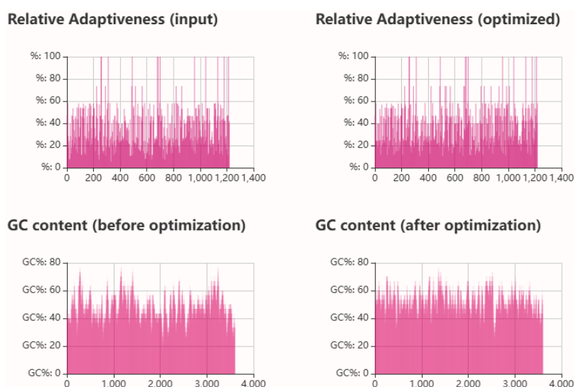
شکل ۷. نمودارهای بهینه‌سازی و محتوای GC پروتئین کایمر، پیش و پس از بهینه‌سازی
