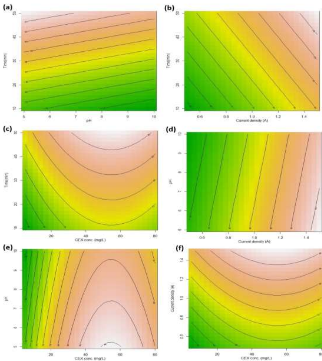
شکل ۳. نمودار کانتور بازده حذف آموکسی سیلین، به عنوان تابعی از برهم کنش زمان (دقیقه)، pH، دانسیته ی جریان ( \text{mA}/\text{cm}^2 ) و غلظت آموکسی سیلین (میلی گرم در لیتر) در مرکز (بهینه) سایر پارامترها
