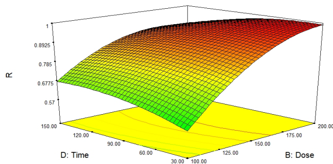
شکل ۱۰: برهمکنش اثر زمان تماس و دوز نانوکاتالیست در حذف DEP با استفاده از GO-ZnO/LED (pH برابر ۷ و غلظت اولیه جاذب ۱۰ میلی گرم بر لیتر)
