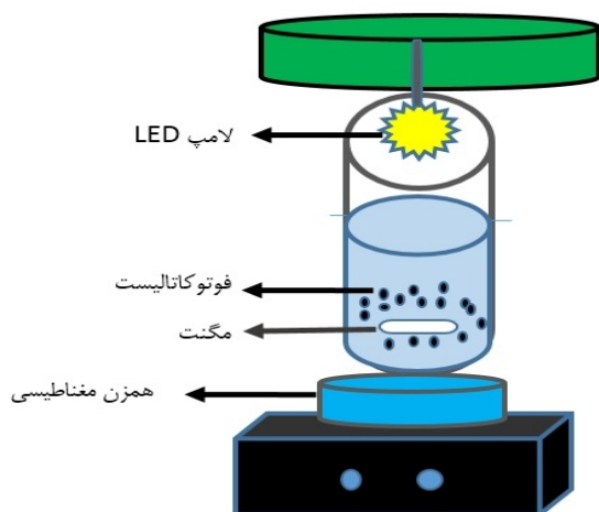
شکل ۱: شماتیک پایلوت سیستم ناپیوسته مورد استفاده در تحقیق
