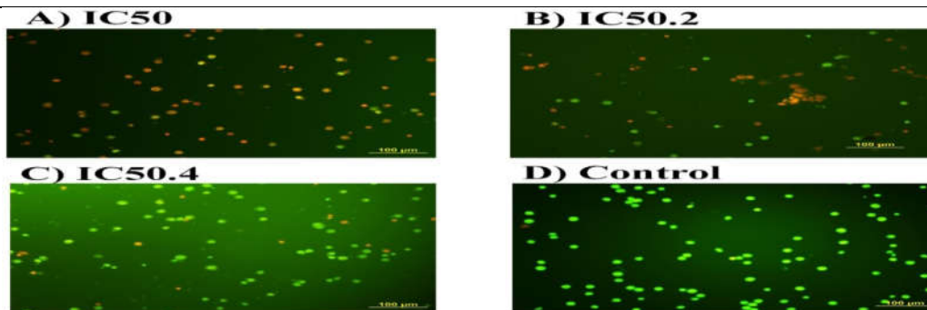
شکل ۱. رنگ آمیزی آکریدین اورنج / اتیدیوم بروماید برای سلول‌های HL-60 در غلظت‌های مختلف مرزنجوش. مراحل آپوتوز اولیه و ثانویه و نکروز در سلول‌های تیمار شده با مقادیر (A) برابر، (B) نصف و (C) ۱/۴ از مقدار IC50 ۷۲ ساعته مرزنجوش با رنگ آمیزی آکریدین اورنج / اتیدیوم بروماید نشان داده شد. در این رنگ آمیزی سلول‌ها ۴ دسته می‌شوند: سلول‌های یکنواخت سبز رنگ، سلول‌های سالم می‌باشند؛ سلول‌های سبز رنگ با هسته قطعه قطعه، در مرحله آپوتوز اولیه می‌باشند؛ سلول‌های نارنجی رنگ با هسته قطعه قطعه، در مرحله آپوتوز تأخیری و سلول‌های یکنواخت نارنجی رنگ، سلول‌های نکروتیک در نظر گرفته می‌شوند. در بخش A، سلول‌هایی با هسته نارنجی رنگ یکنواخت و قطعه قطعه زیادند که نشان دهنده نکروتیک و آپوتوتیک تأخیری بودن سلول‌ها می‌باشند. در بخش B، علاوه از سلول‌های مرحله A، سلول‌های سبز رنگ با هسته قطعه قطعه زیاد مشخص شده‌اند که نشان می‌دهد از میزان آپوتوز کاسته شده است. در بخش C، علاوه از سلول‌های نکروتیک و آپوتوتیک، سلول‌های سالم نیز مشاهده می‌شوند. در بخش D، سلول‌های سبز رنگ یکنواخت نشان دهنده سالم بودن سلول‌ها است. استفاده شونده در درمان لوسمی پرومیلوسیت حاد می-باشند (۲۷).
