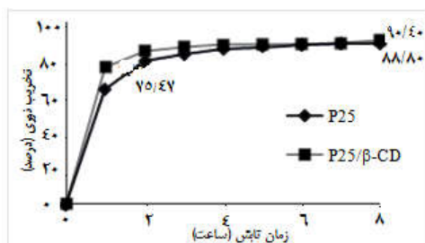
شکل ۸. تخریب نوری ۴۲-دی کلرو فنوکسی استیک اسید (۲۰ mg/L) با نانو نور کاتالیز گر P25 (۵۰۰ mg) و P25/β-CD (۵۵۰ mg) در راکتور نوری با جریان پیوسته (منبع تابش: مجموع LED ها با توان ۱۰۰ وات، طول موج ۳۶۵ نانومتر و شدت جذب ۱۰۰ mW/cm)
