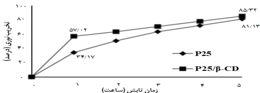
شکل ۷. تخریب نوری ۴۲-دی کلروفنوکی-استیک اسید (۲۰ mg/L) با نانو نور کاتالیز گر P25 (۵۰ mg) و P25/β-CD (۵۵ mg) در راکتور نوری با جریان ناپیوسته (منبع تابش: LED با توان ۲۰ وات، طول موج ۴۰۰ نانومتر و شدت جذب ۱۰۰ mW/cm)
