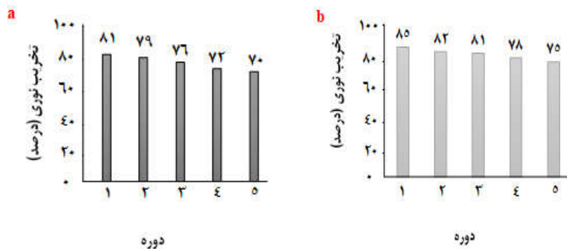
شکل ۹. بازیافت و کارایی نور کاتالیز گر (a) P25، (b) P25/β-CD در تخریب نوری ۴۲-دی کلرو فنوکسی استیک-اسید در محلول های آبی با لامپ LED با توان ۲۰ وات و طول موج ۴۰۰ نانومتر با شدت جذب ۱۰۰ mW/cm بعد از ۵ دوره در راکتور نوری با جریان ناپیوسته
