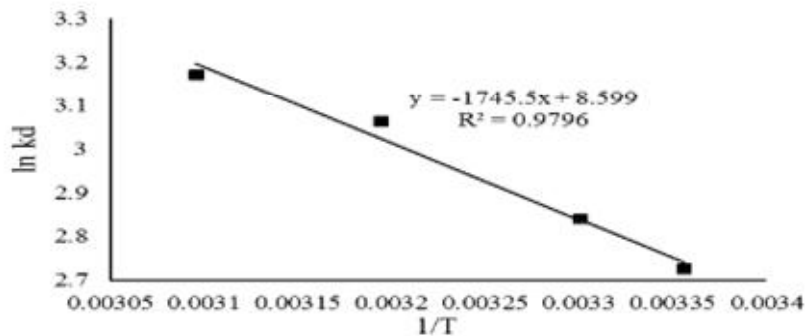
شکل ۱۳: نمودار Van,t Hoff Curve برای کلرپیریفوس روی CGO
