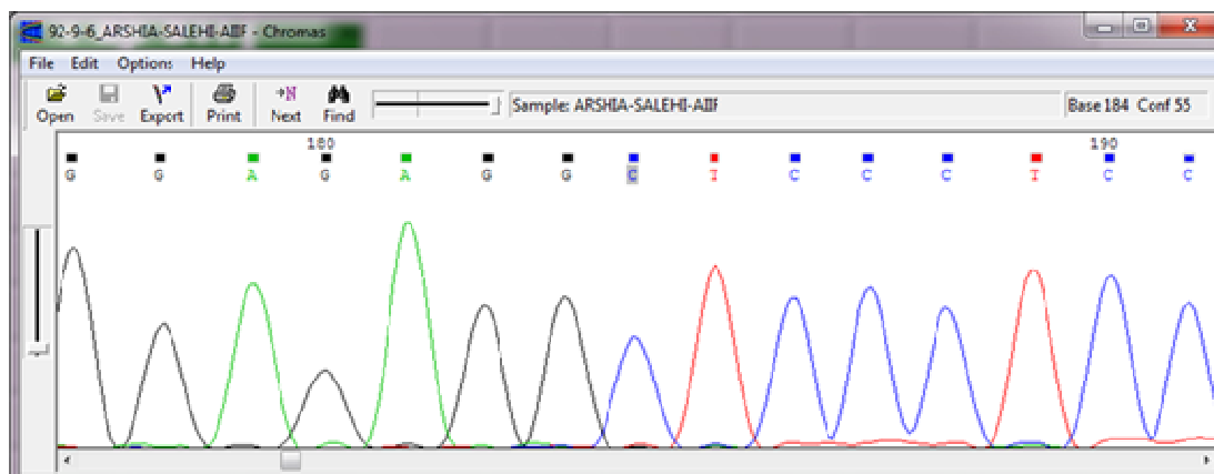
شکل ۱- جهش نقطه ای ( \alpha 5nt ): در محل مشخص شده توالی TGAGG حذف شده - ->GAG GTG AGG (GAG GTG AGG>GAG G- -) که با توجه به وجود یک حذف بزرگ در کروموزوم دیگر، در الکتروفوروگرام به صورت هموزیگوت مشاهده می شود.
