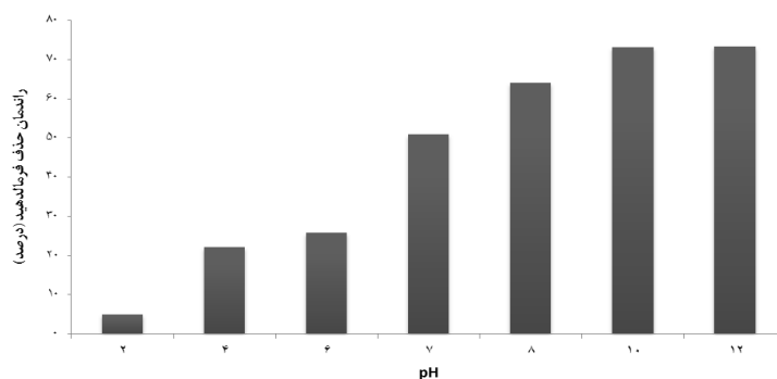
نمودار ۲- راندمان حذف فرمالدهید در pH های متفاوت توسط فرآیند الکتروفنتون ( C_0=7500\text{mg/L} , I=8.5\text{mA/cm}^2 , \text{H}_2\text{O}_2=50\text{mM/L} , t=10\text{min} , V=200\text{cc} )
