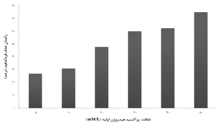
نمودار ۳- راندمان حذف فرمالدهید در غلظت های متفاوت هیدروژن پراکسید توسط فرآیند الکتروفنتون: ( C_0=7500\text{mg/L} , I=8.5\text{mA/cm}^2 , \text{pH}=10 , t=10\text{min} , V=200\text{cc} )
