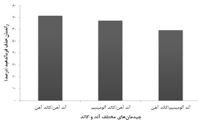
نمودار ۴- راندمان حذف فرمالدهید توسط فرآیند الکتروفنتون حین استفاده از الکترودهای مختلف: ( C_0=7500\text{mg/L} , t=10\text{min} , I=8.5\text{mA/cm}^2 , \text{pH}=10 , \text{H}_2\text{O}_2=50\text{mM/L} , V=200\text{cc} )
