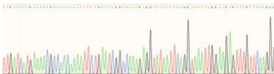
شکل ۹. بخشی از نتیجه توالی یابی cDNA فاکتور ۹ انسانی کلون شده در پلاسمید نوترکیب pcDNA3-hFIX-EGF با استفاده از پرایمر رفتی hFIX-EcoRI .
