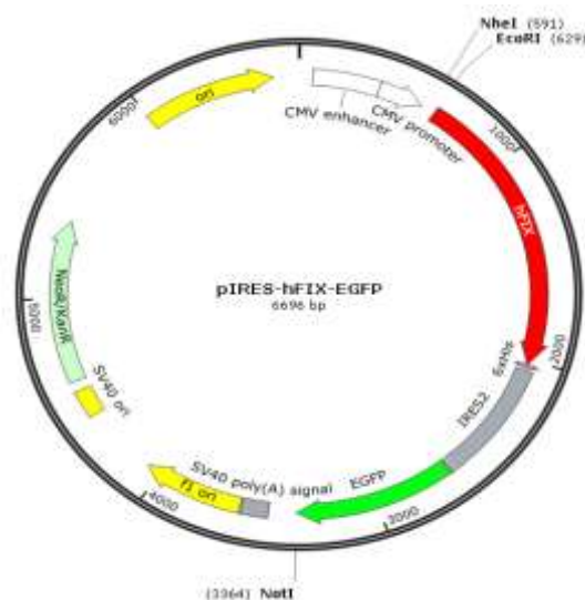
شکل ۲. شکل شماتیک از پلاسمید دو سیستمی نوترکیب pIRES-hFIX-EGFP.
