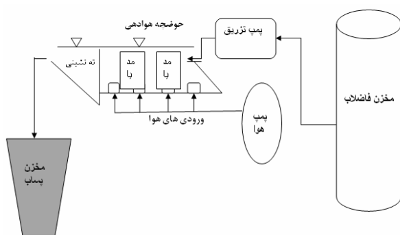
شکل ۱: نمای شماتیک راکتور لجن فعال دارای بستر ثابت رشد میکروب
