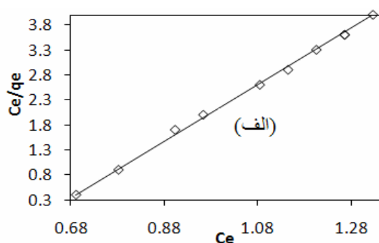
نمودار ۴: مدل ایزوترمی لانگمویر (الف) و فروندلیخ (ب) بر روی کارایی حذف
