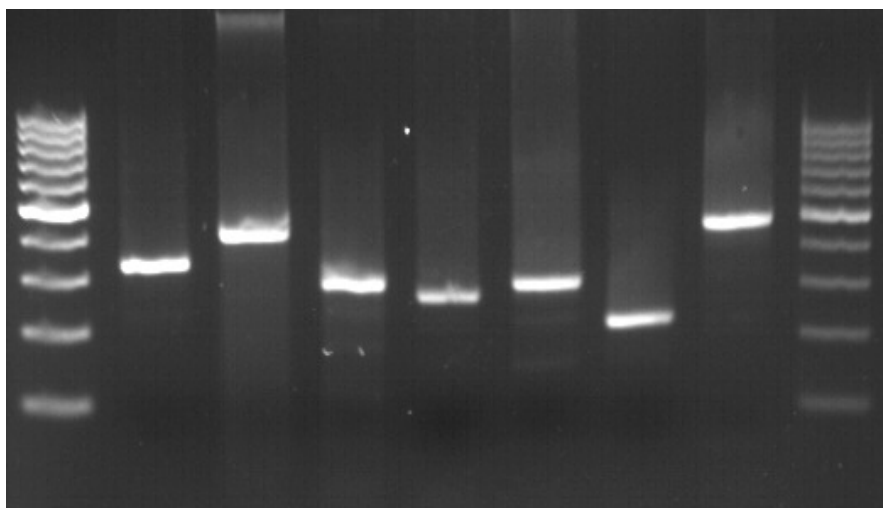
شکل ۱: VNTR لوکوس‌ها به ترتیب A-ETR-ETR-F, ETR-B, ETR-C, ETR-D, ETR-E در سویه استاندارد H 37 RV
