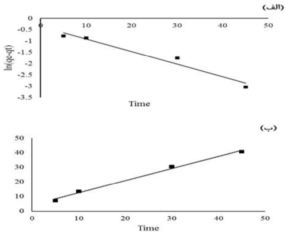
شکل ۱۱: نمودار شبه سینتیک درجه اول (الف) شبه سینتیک درجه دوم (ب) برای جذب کلرپیرفوس روی کیتوزان گرافن اکساید
