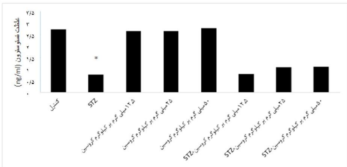
نمودار ۱. تاثیر غلظت‌های مختلف کروسین و STZ بر میزان هورمون تستوسترون در گروه‌های مورد مطالعه P = 0.000 * در گروه دریافت کننده STZ در مقایسه با گروه کنترل p < 0/05 در گروه دریافت کننده همزمان STZ و کروسین در مقایسه با گروه دریافت کننده STZ
