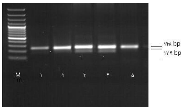
شکل ۳: الکتروفورز قطعه ۲۴۸bp و ۱۷۴ bp ستون ۱، H37RV و ستونهای ۲ و ۵ عدم موتاسیون و ستونهای ۳ و ۴ دارای موتاسیون در لوکوس inhA(-15C → T)، مارکر ۱۰۰ b
