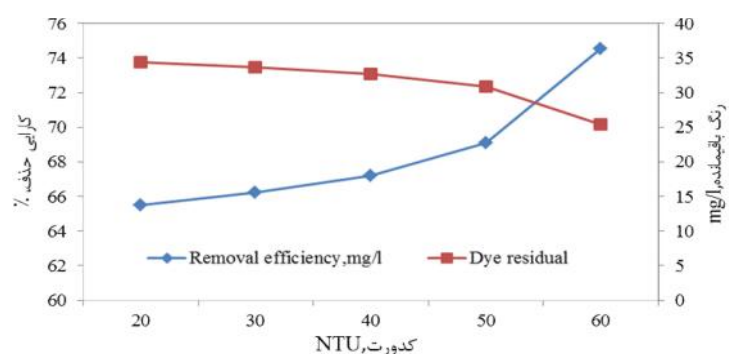
نمودار ۳: تاثیر کدورت در کارایی حذف رنگ راکتیو قرمز ۱۹۸ از محلول سنتتیک (غلظت رنگ = ۵۰ میلی گرم در لیتر، pH=۱۲، دوز منعقد کننده = ۳ ml/L)
